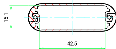
A-A (1:1)
